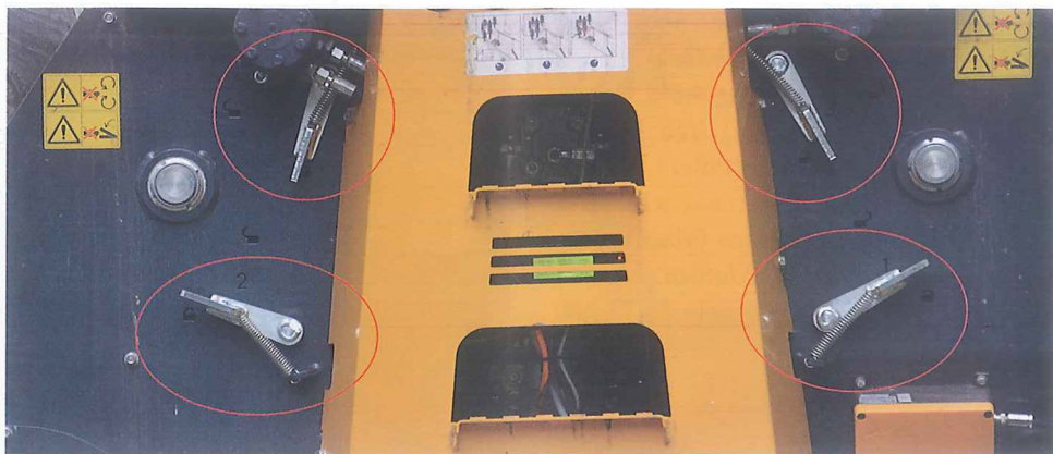
Ročno varovanje- zaklep (označeno z rdečimi krogi) sidrnih vrvi.
