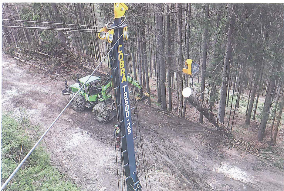
Prihod vozička na zgornjo postajo.
